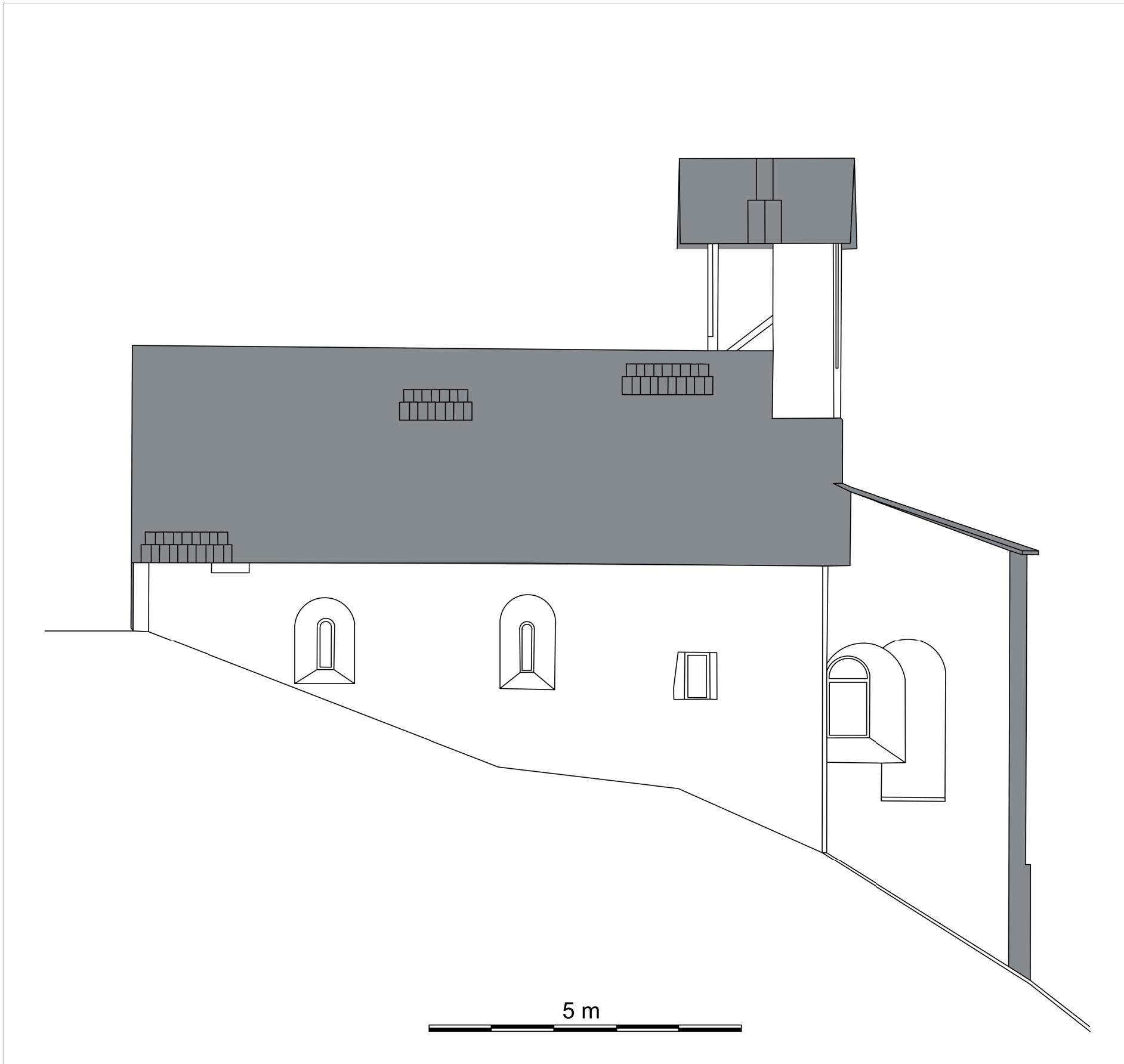
Plan 3: St. Stephan ob Burgeis. Ansicht der Südfassade. Zeichnung nach Iris Federspiel und Joerg Willich.
